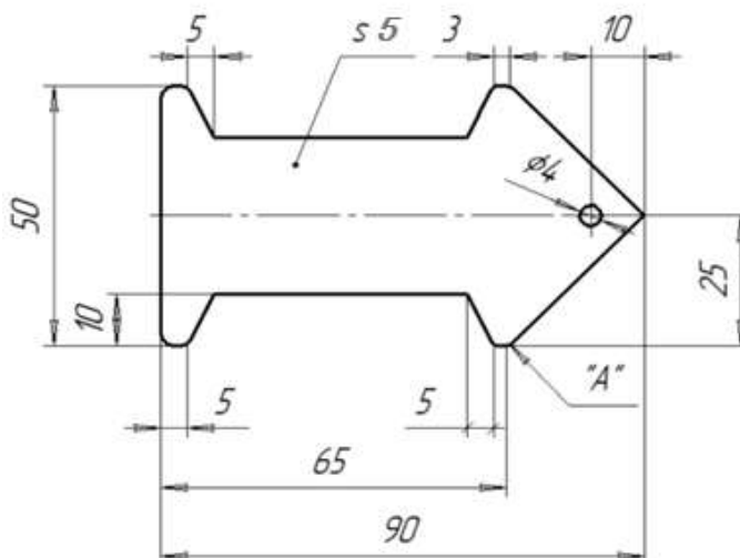
Рис. 2. Чертёж бобины для ниток
